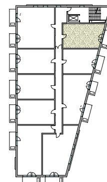
MIESZKANIE M-20 ( PIĘTRO II) SKALA 1:70
